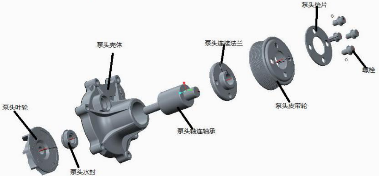
S500L1-1307100泵头分解图
